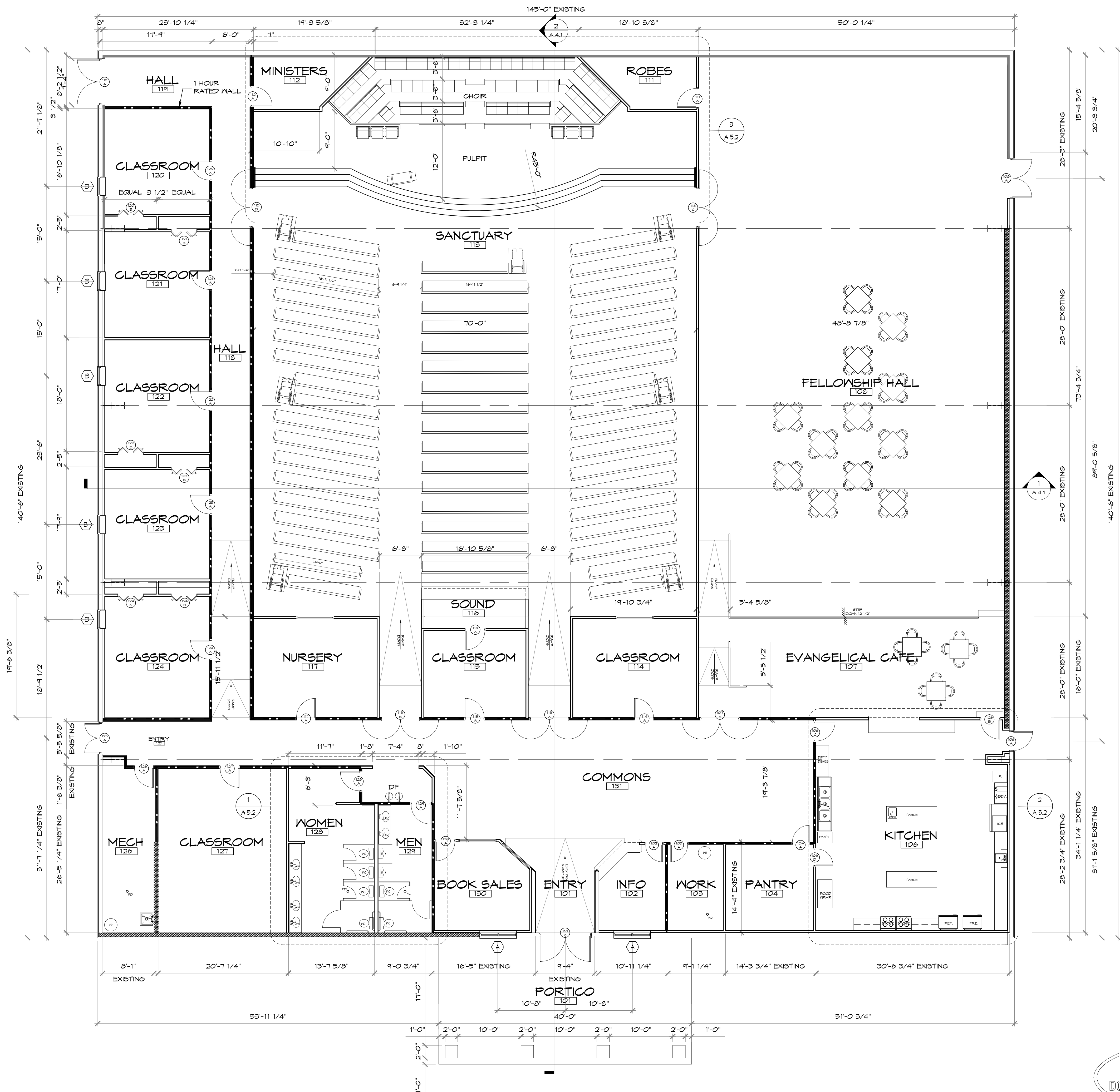
FLOOR PLAN SCALE: 1/8" = 1'-0"
